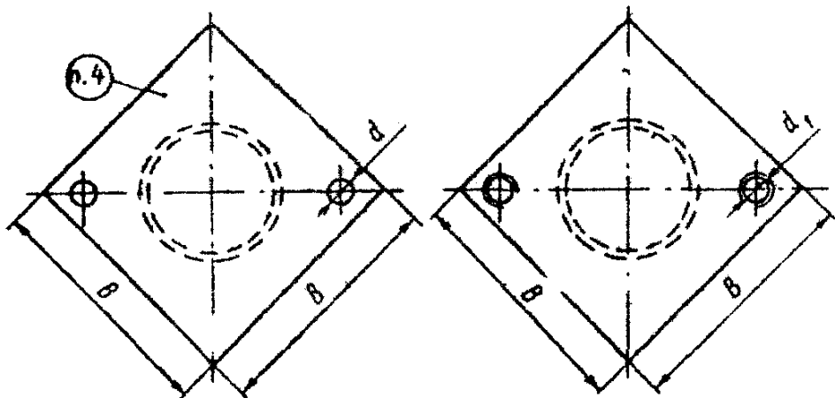
Вид А
