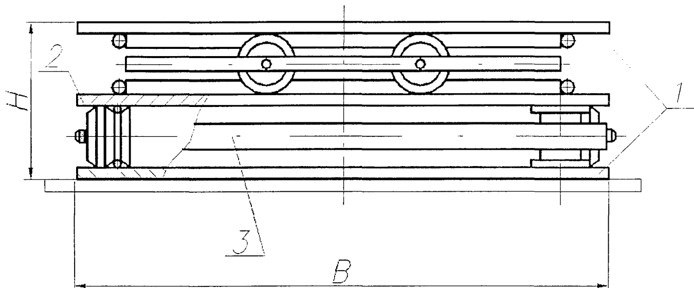
1 – опорная плита; 2 – промежуточная опорная плита; 3 – катковая обойма
